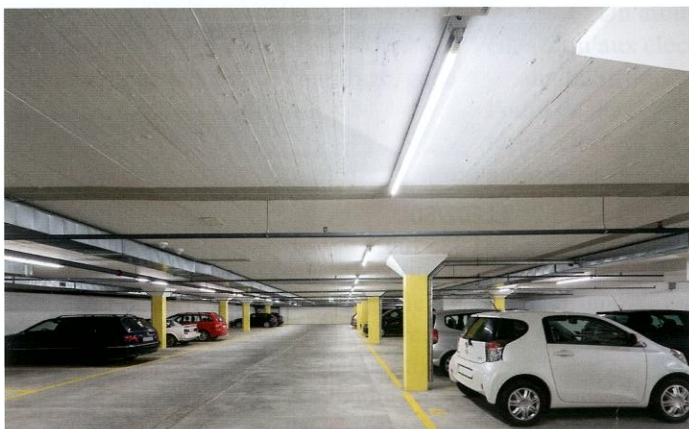
Der Einsatz von LED-Tubes in einer Autoeinstellhalle bzw. in einer Autoausstellung ermöglicht erhebliche Energieeinsparungen.
